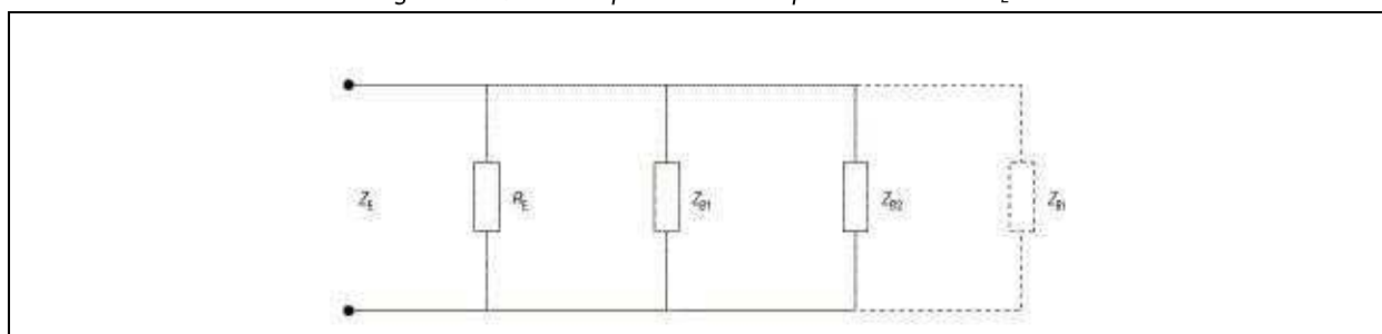
Figure 2.9. Schéma équivalent de l'impédance de terre Z_E
