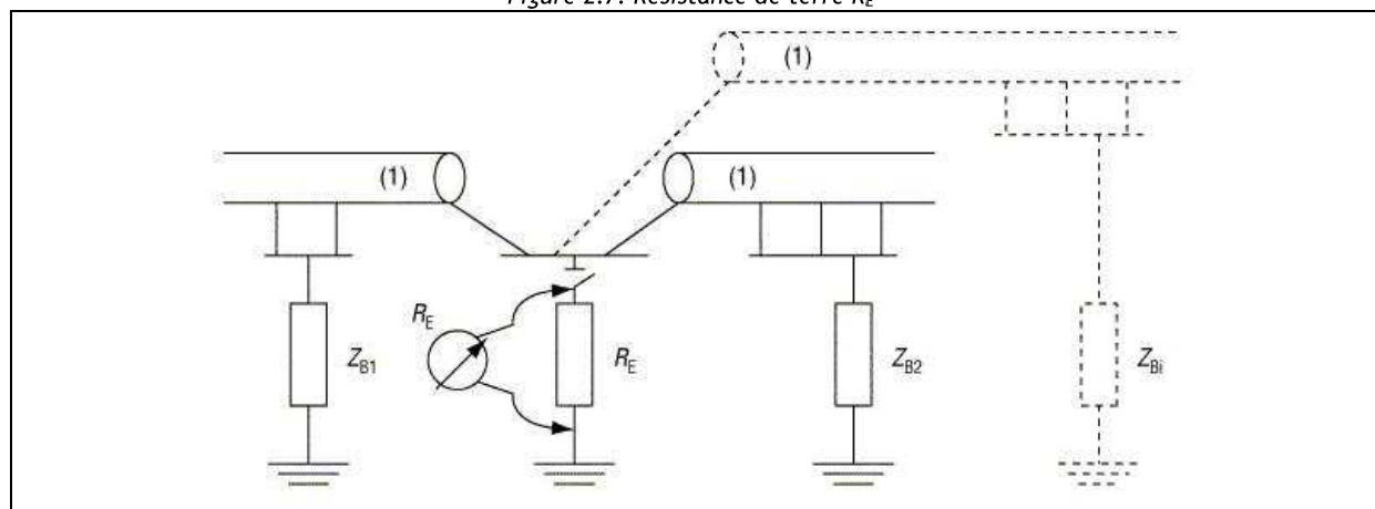
Figure 2.7. Résistance de terre R_E
