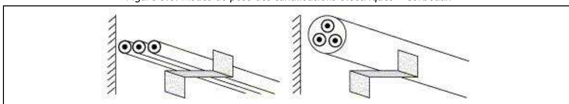
Figure 5.6. Modes de pose des canalisations électriques – Corbeaux
